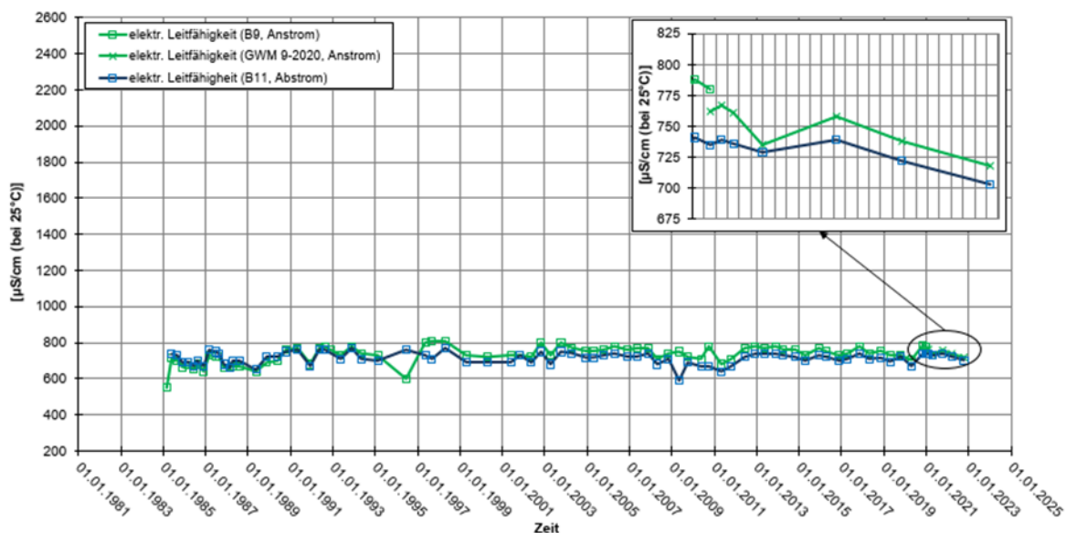
Abb. 2-1: Leitfähigkeiten im Anstrom (B9 ab Ende 2020 GWM9/2020) und Abstrom (B11) der SAD Rondeshagen
